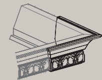
CAPITELLO ANGOLO ESTERNO EXTERNAL CORNICE DECORATION 227,2 x 227,2 x 107,2
